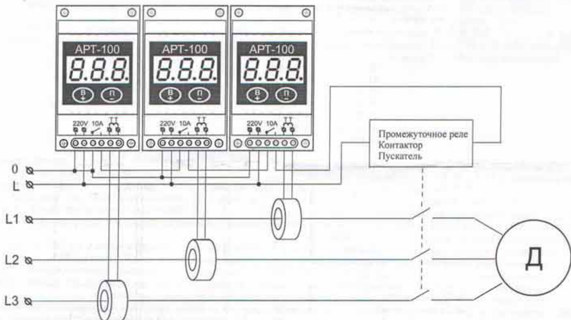
Рис.2 Вариант защиты по току трехфазного потребителя.
