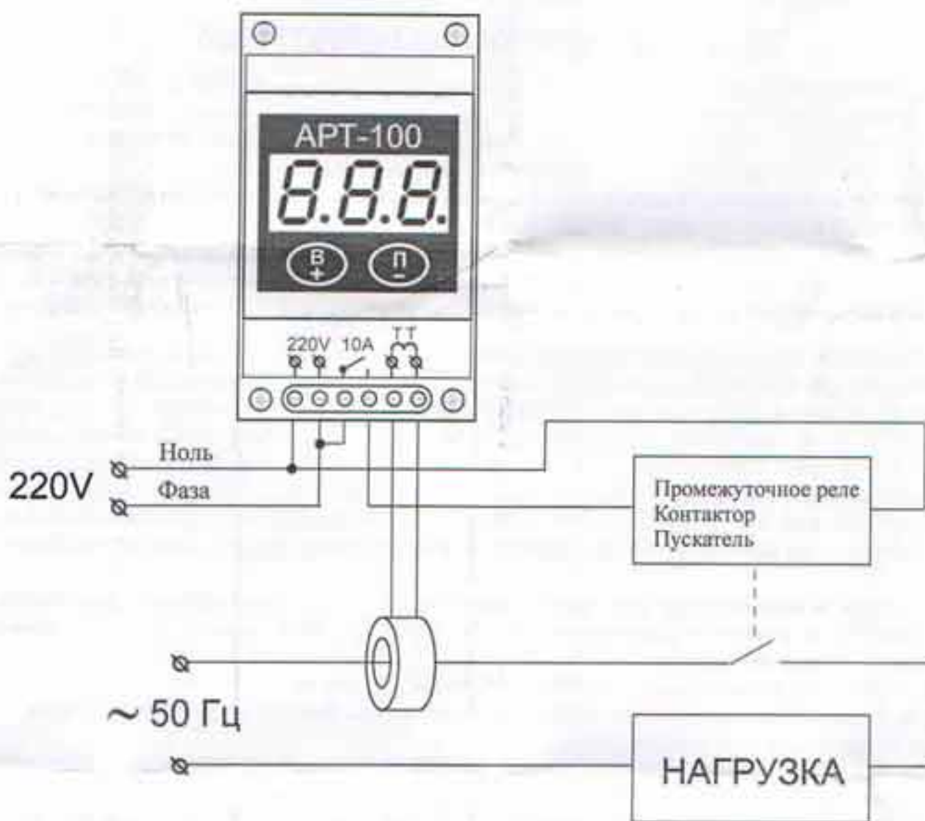
Рис.1 Вариант подключения прибора.
