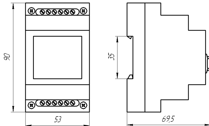
Рисунок 1 - Габаритные и установочные размеры реле
